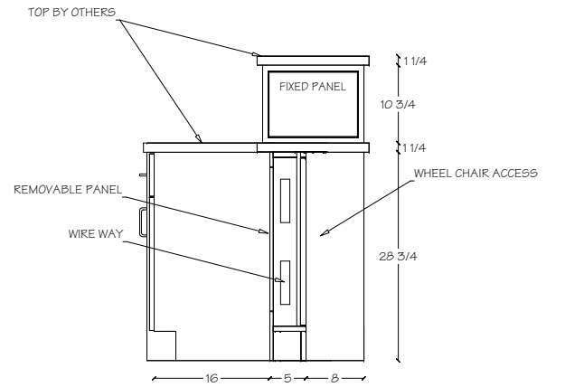
E Section (Center) Scale: 1/2=1
