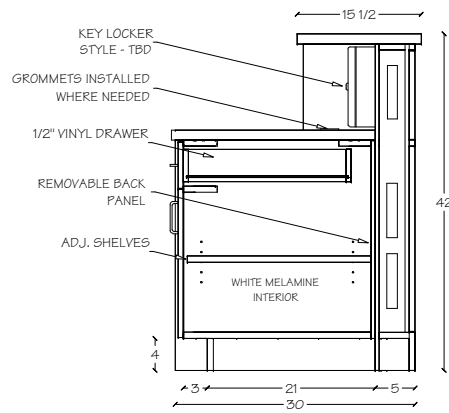
F Section (Cabinet) Scale: 1/2=1
